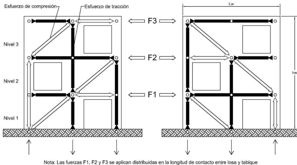
Figura 3.13. Modelo biela-tirante para tabiques poco esbeltos con aberturas dispuestas en forma irregular.
