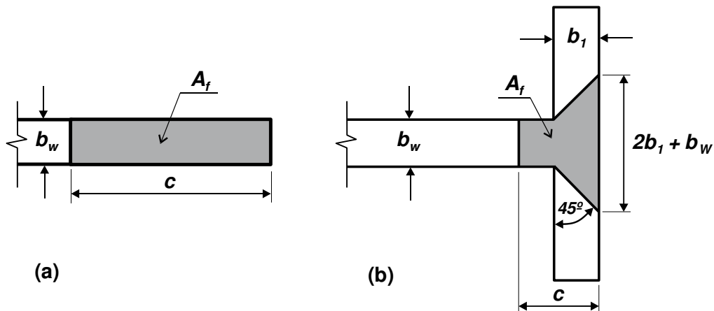
Figura 3.10. Área efectiva para determinar la fricción por corte.
