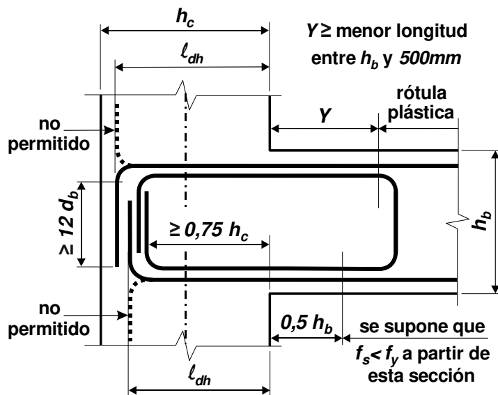
Figura 2.8. Anclaje de la armadura longitudinal de una viga cuando la sección crítica de formación potencial de rótula plástica está a una distancia de la cara de la columna de al menos la altura de la viga o a 500 mm.
