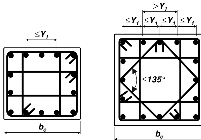
Figura 2.17. Detalles de armadura transversal de columnas rectangulares en zona de rótula plástica.
