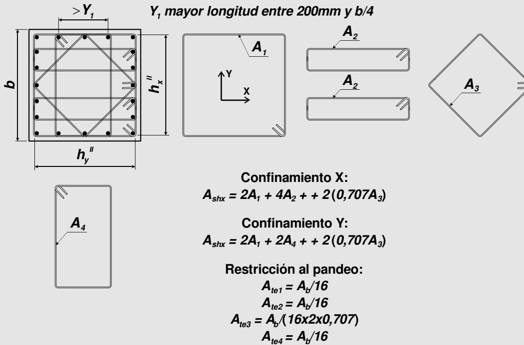
Figura C2.10. (continuación) Ejemplos de disposición de armadura transversal en zona de rótula plástica en una columna cuadrada, considerando que f_y = f_{yt} , y una separación s = 6d_b .
