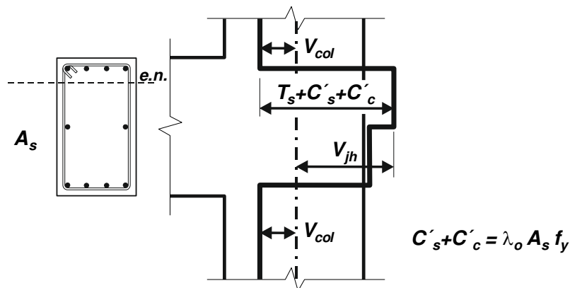
Figura 2.23. Corte horizontal en un nudo externo, con viga armada convencionalmente.
