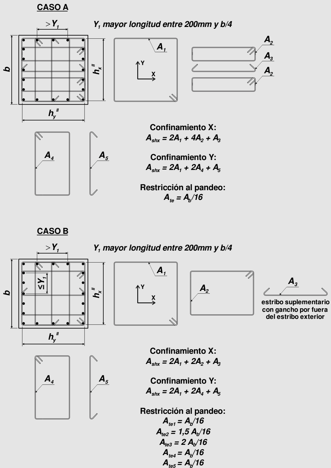
Figura C2.10. Ejemplos de disposición de armadura transversal en zona de rótula plástica en una columna cuadrada, considerando que f_y = f_{yt} , y una separación s = 6d_b .
