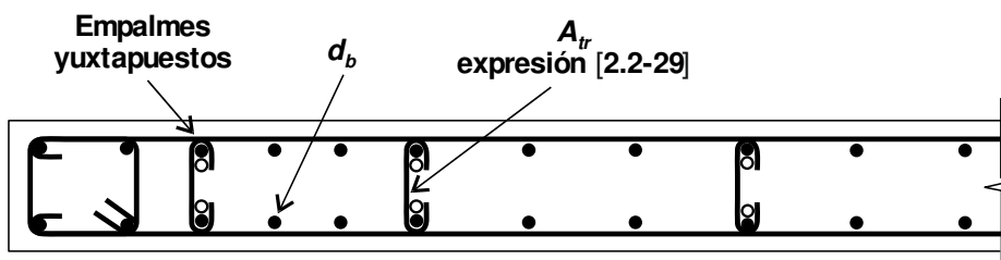
Figura 3.7. Estribos requeridos en empalmes por yuxtaposición.
