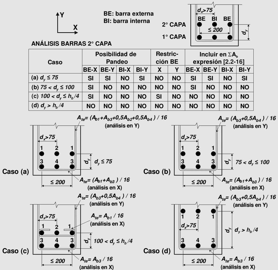
Figura C2.3. Restricción al pandeo de una segunda capa de barras longitudinales, considerando que f_y = f_{yt} , y una separación s = 6d_b .
