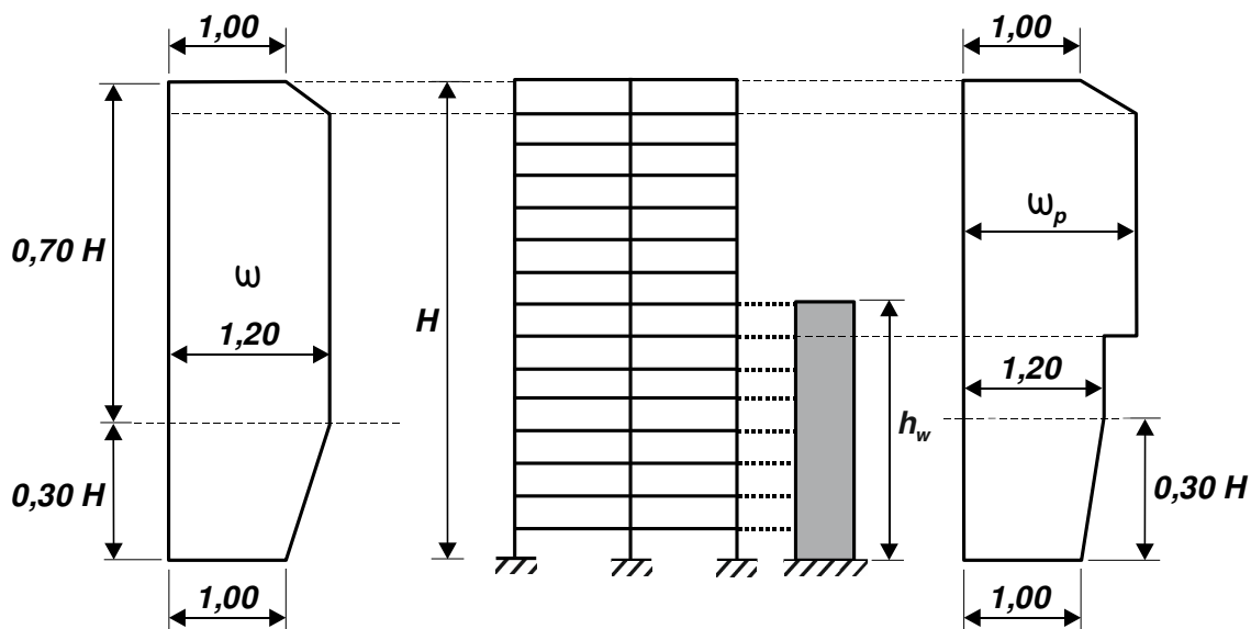
(a) Tabique sismorresistente con altura h_w total
