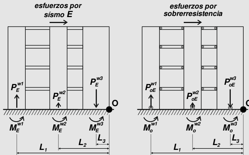
Figura C3.8. Factor de sobrerresistencia para un sistema de tres tabiques acoplados.
