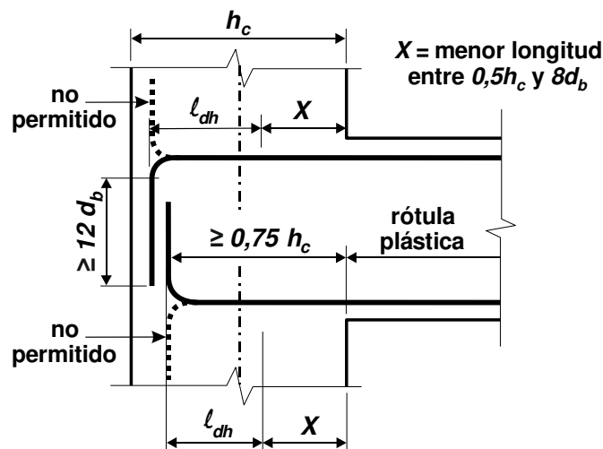
Figura 2.7. Anclaje de la armadura longitudinal de una viga cuando la sección crítica de formación potencial de rótula plástica está en la cara de la columna.
