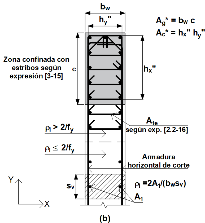
Figura 3.6. Zonas de armadura transversal de acuerdo con el artículo 3.5.6.
